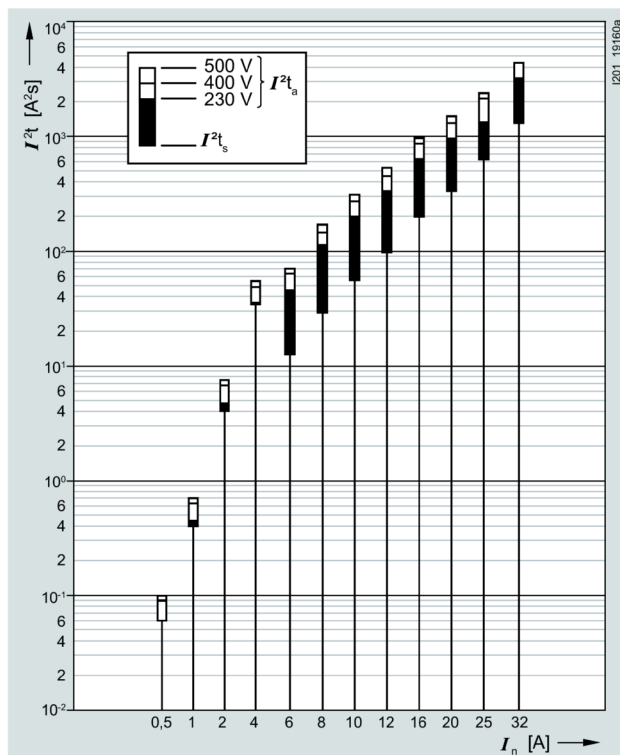
Melting I^2t values diagram
