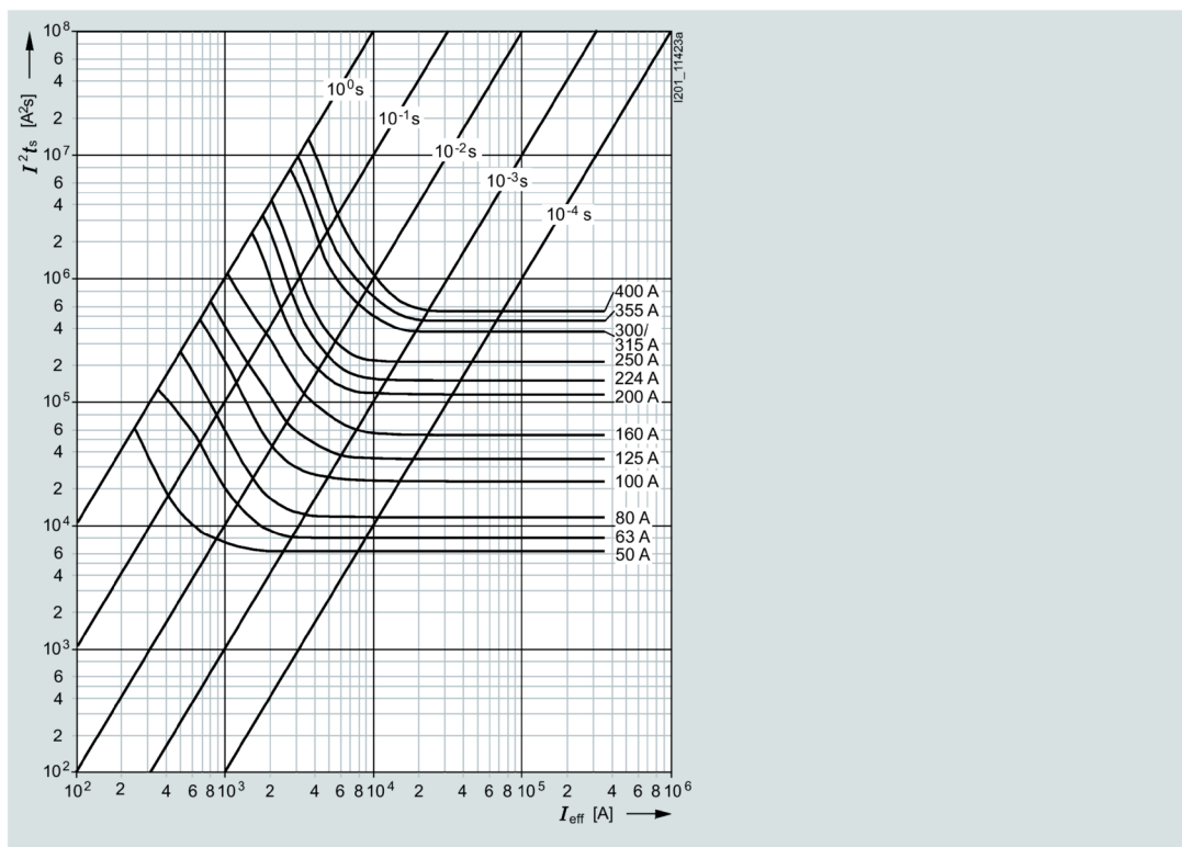
Melting I^2t values diagram
